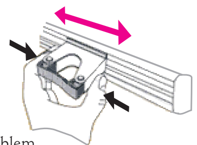
Alu - Geräteleiste 500 mm, komplett mit 9 Haken, glasfaserverstärkt, verschiebbar, Hakenfarbe weiß o. blau (Beispielabbildung)
